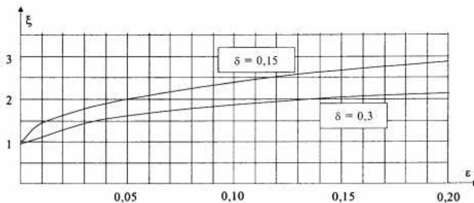
Рисунок 11.1 – Коэффициенты динамичности
